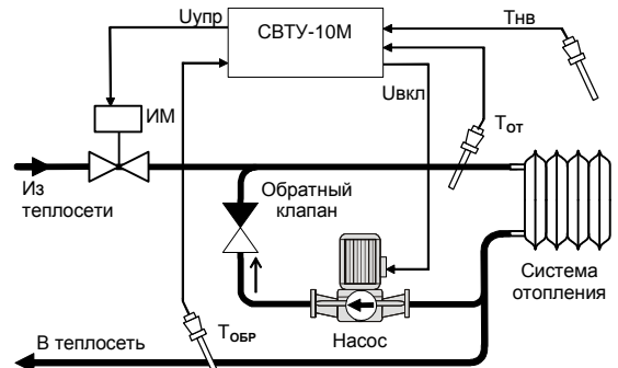
Рис.6 Регулирование температуры на выходе контура отопления с коррекцией по Тнв
