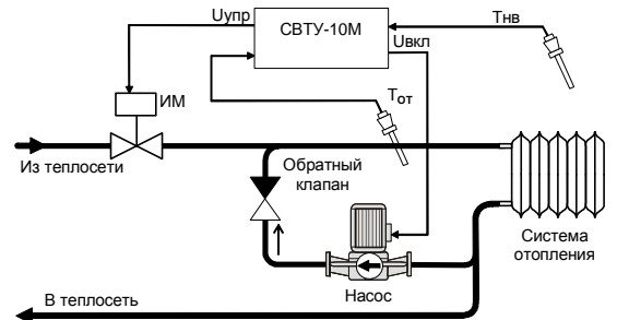
Рис.4 Регулирование температуры на входе контура отопления с коррекцией по Тнв
